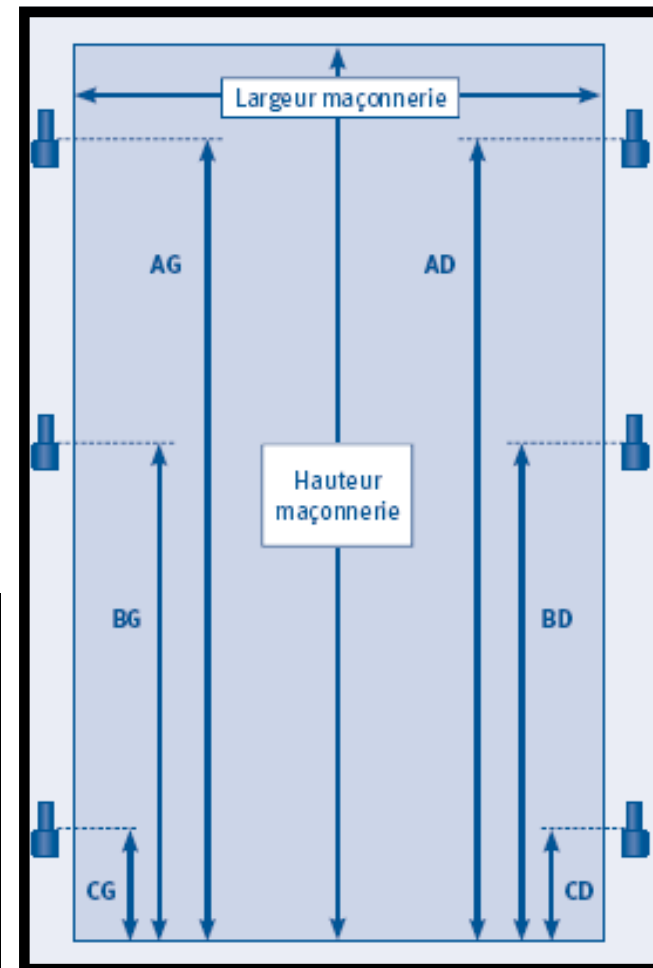
C : Du bas de la maçonnerie au bas de la penture.
